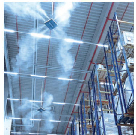
Hochdruck-Luftbefeuchter DRAABE TurboFogNeo 8 im Hochregallager
